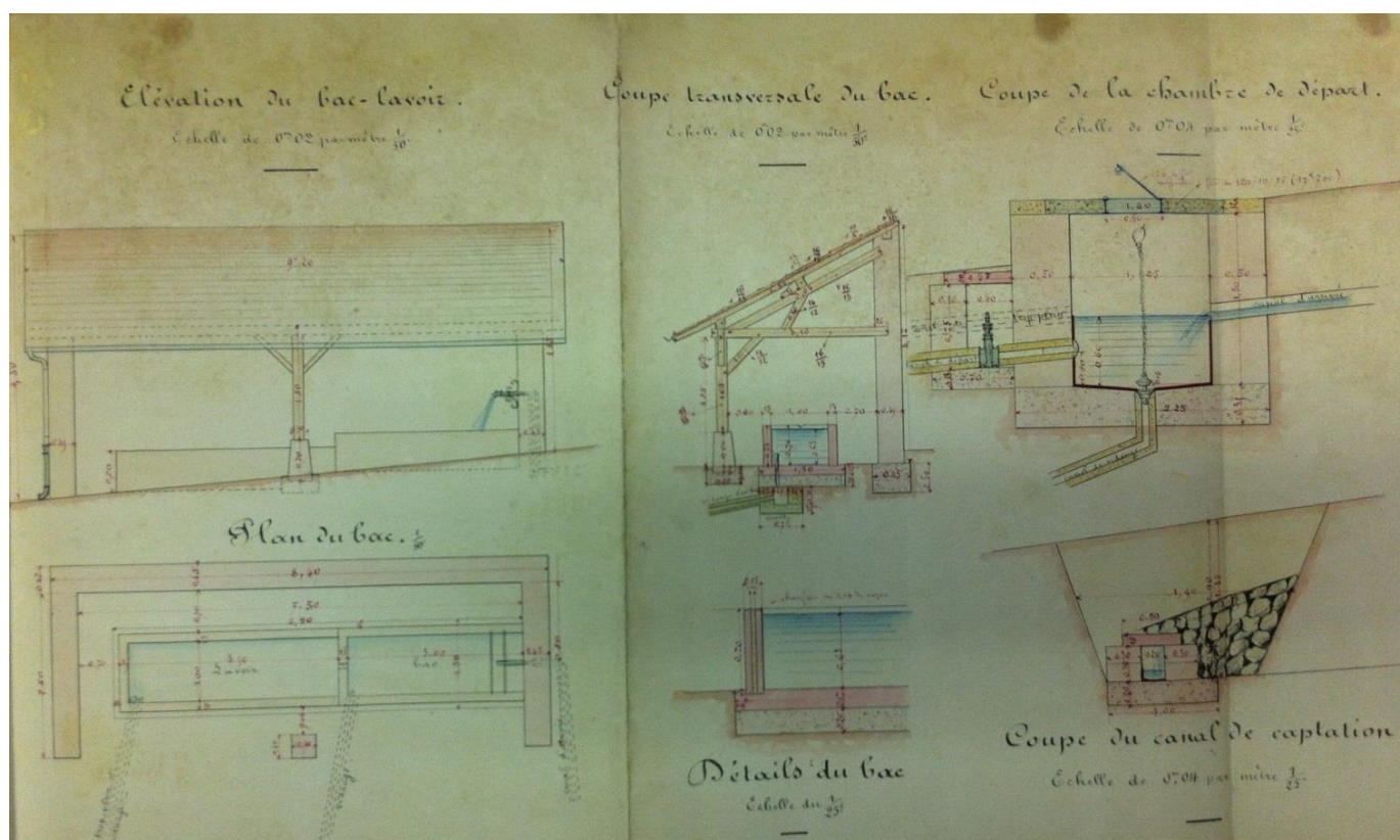
Figure 1 - Plan du lavoir de Craz, M4 (1877).
