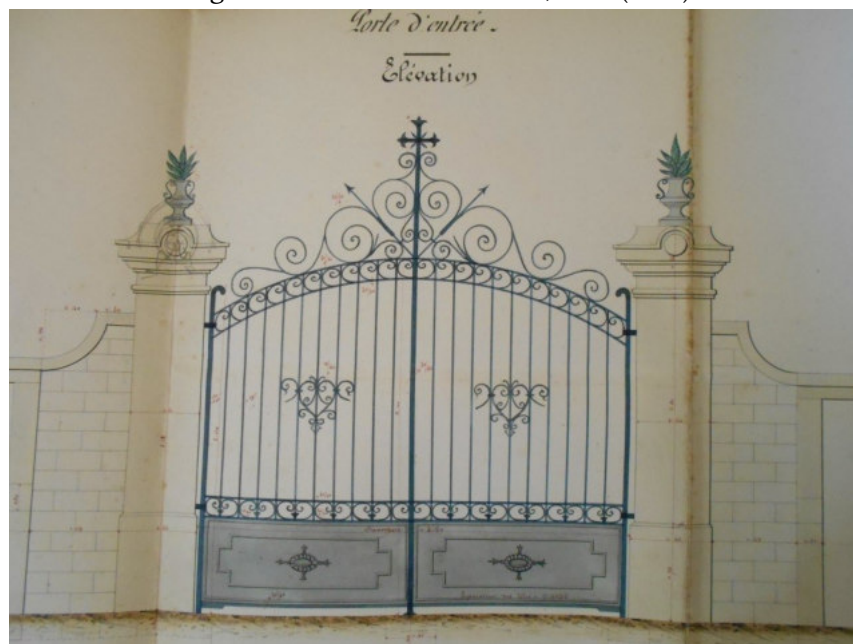
Figure 4 - Dessins des portes principales pour le projet d'agrandissement du cimetière, M11 (1886).
